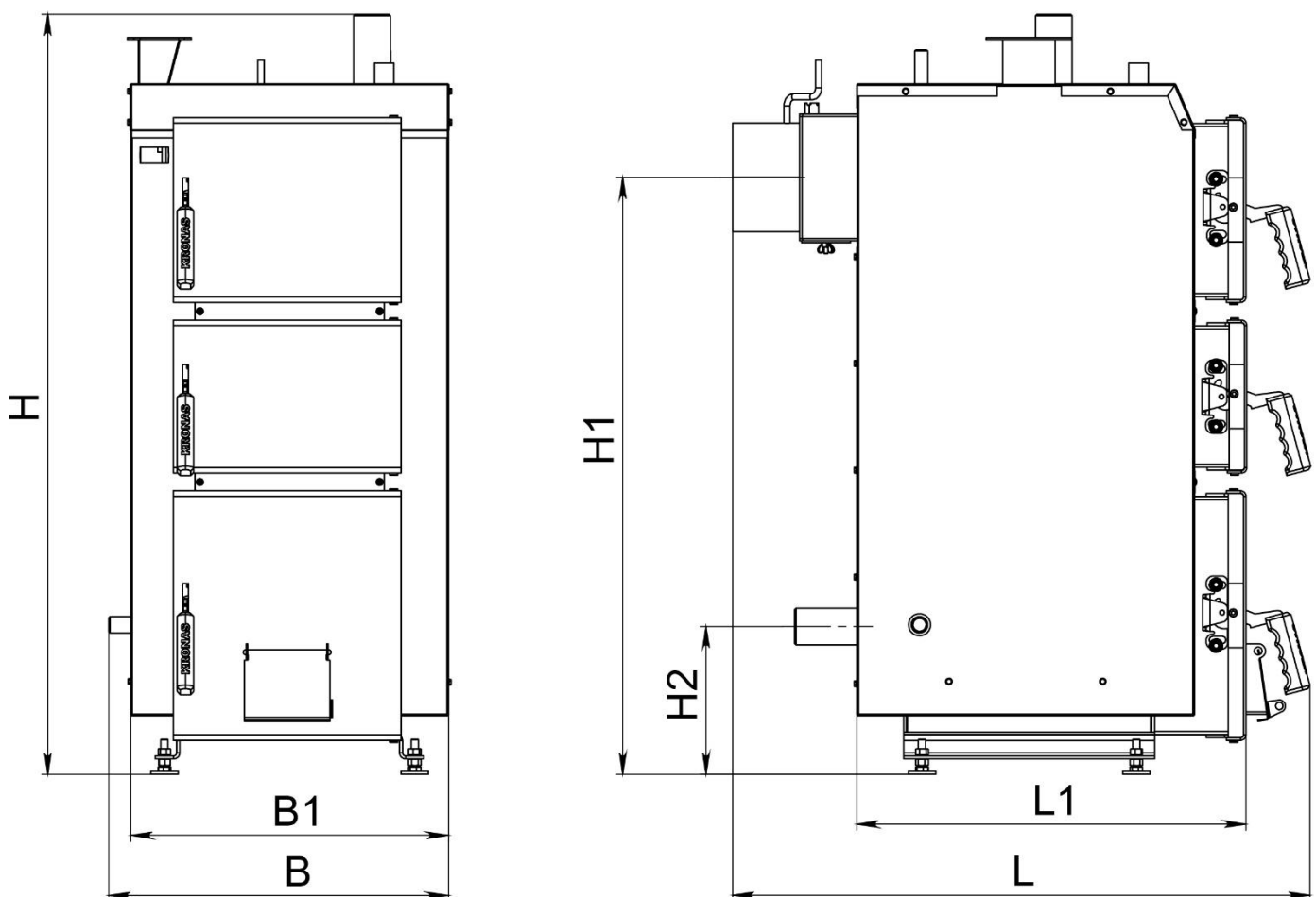
Рисунок 3.1 – Позначення габаритів котла типу К (потужністю 15-30 кВт)
